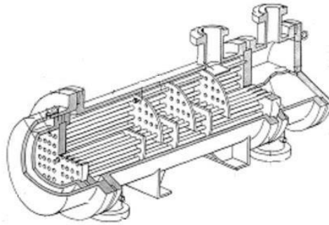
Ilustración 36. Evaporador de Carcasa y Tubos. [40]
