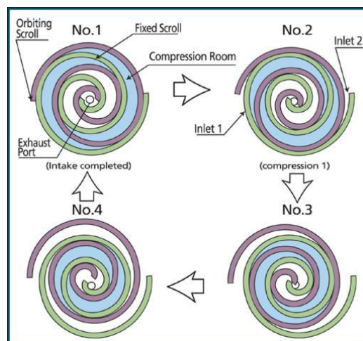
Ilustración 30. Proceso Compresor Scroll.[33]
